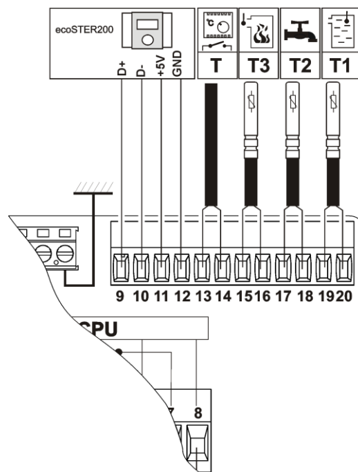
Rys. 12 Schemat połączeń elektrycznych z urządzeniami zewnętrznymi, wykonanie ES , gdzie: T1 - czujniki temperatury kotła (typ CT4), T2 - czujniki temperatury ciepłej wody użytkowej (typ CT4), T3 - czujnik temperatury spalin (typ CT2s, CT2s-2), T - standardowy termostat pokojowy, TIS TRONIC 297 - panel pokojowy z funkcją termostatu pokojowego.
