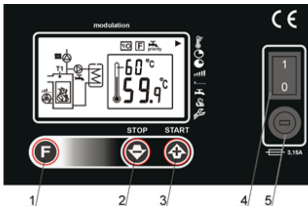
Rys. 1 Widok klawiatury
