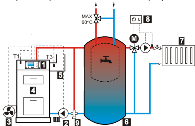
Rys. 7 Schemat hydrauliczny z buforem cieplnym, gdzie: 1 – regulator, 2 – pompa centralnego ogrzewania, 3 – wentylator, 4 – kocioł, 5 – przewód kominowy, 6 – bufor ciepły ze zintegrowanym zasobnikiem ciepłej wody użytkowej, 7 – instalacja centralnego ogrzewania, 8 – regulator zewnętrzny obiegu grzewczego, 9 – zawór termostatyczny chroniący powrót kotła, T1 – czujnik temperatury kotła, T3 – czujnik temperatury spalin (opcjonalnie, nie jest wymagany do normalnej pracy).
