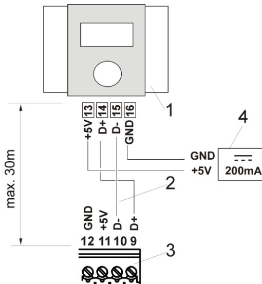
Rys. 15 Podłączenie panelu pokojowego TIS TRONIC 297 – dwuprzewodowe, gdzie: 1 – TIS TRONIC 297, 2 – przewody, 3 – TIS TRONIC 83, 4 – zasilacz 5V min 200mA.
