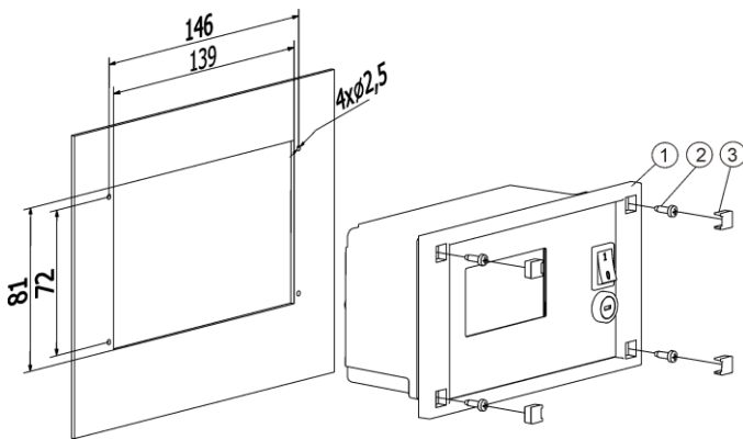
Rys. 8 Zainstalowanie regulatora w płycie montażowej, gdzie: 1 - regulator, 2 - blachowkręt 2.9x9, 3 - zaśleпка.
