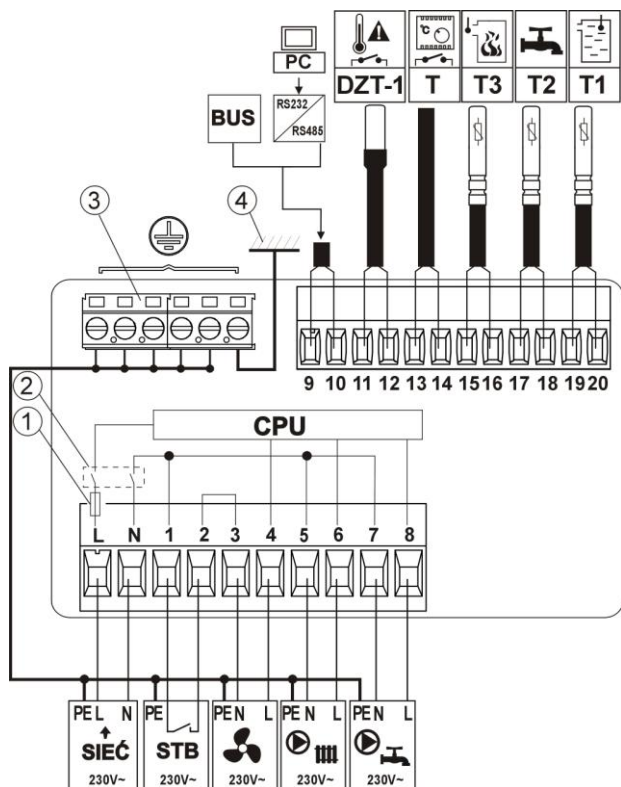
Rys. 11 Schemat połączeń elektrycznych z urządzeniami zewnętrznymi, wykonanie ST. , gdzie: T1 - czujniki temperatury kotła (typ CT4), T2 - czujniki temperatury ciepłej wody użytkowej (typ CT4), T3 - czujnik temperatury spalin (typ CT2s, CT2s-2), T - termostat pokojowy, DZT-1 - dodatkowe zabezpieczenie termiczne (typ DZT-1 85°C lub 90°C), RS232/RS485 - przetwornik, BUS - złącze komunikacji cyfrowej z komputerem (opcja), 1 - bezpiecznik sieciowy w regulatorze, 2 - wyłącznik sieciowy w regulatorze, 3 - zaciski ochronne PE, 4 - metalowa zabudowa regulatora, SIEĆ - przewód sieciowy, STB - ogranicznik temperatury bezpieczeństwa,
