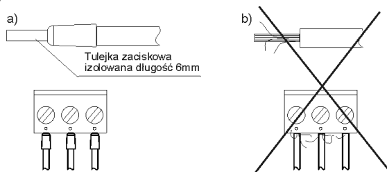
Rys. 13 Zabezpieczanie końców przewodów: a) prawidłowe, b) nieprawidłowe
