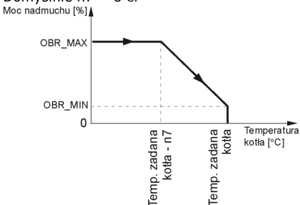
Rys. 17 Redukcja obrotów wentylatora przy regulacji klasycznej
