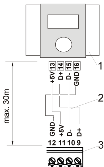
Rys. 14 Podłączenie panelu pokojowego TIS TRONIC 297 – czteroprzewodowe, gdzie: 1 – TIS TRONIC 297, 2 – przewody, 3 – TIS TRONIC 83,
